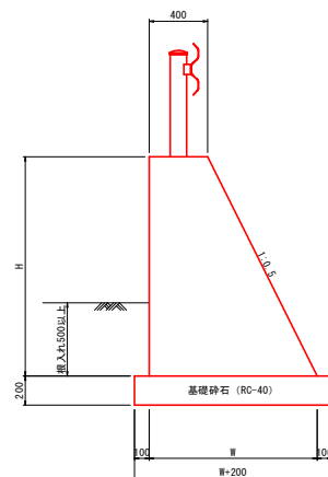
1号重力式擁壁 S=1/20
